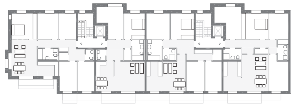
Grundriss 3.OG
