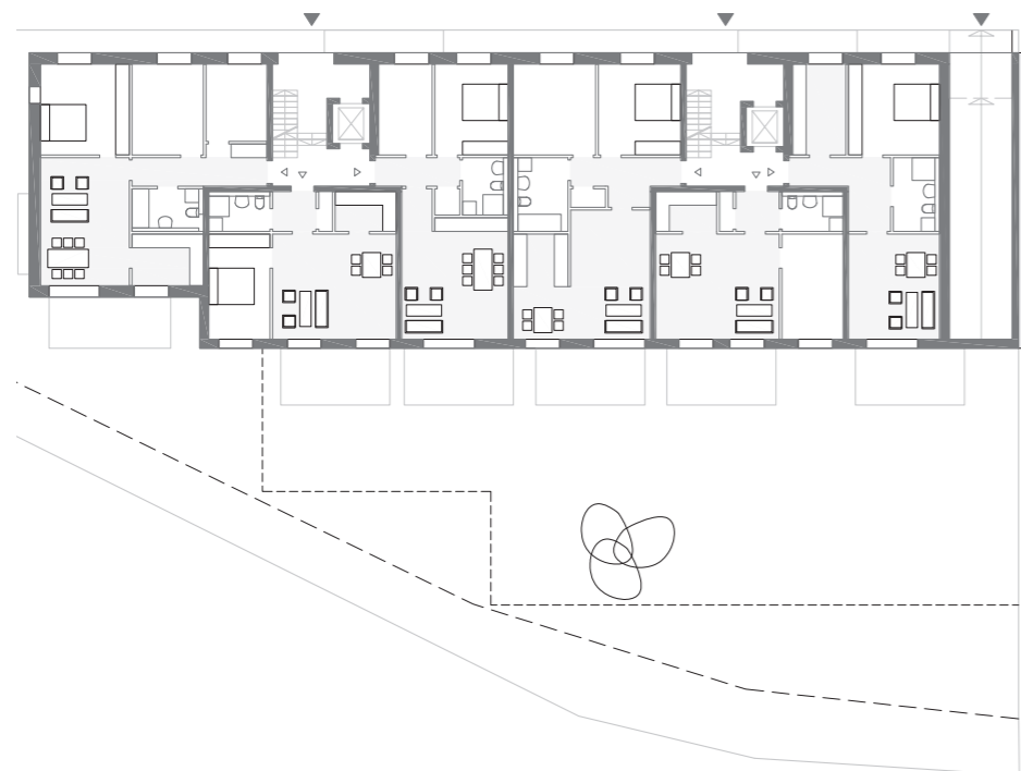
Grundriss 1.+2.OG
